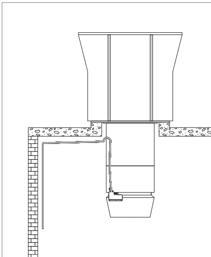
Fig. D15: Condensate line
