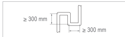
Fig. D11: Oil return trap
