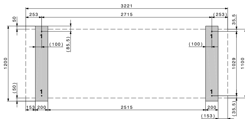
План основи (Размери в mm)
