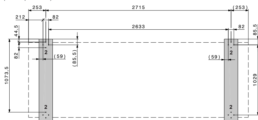
Основният план включва регулируеми крачета за намаляване на вибрациите (Размери в mm)
